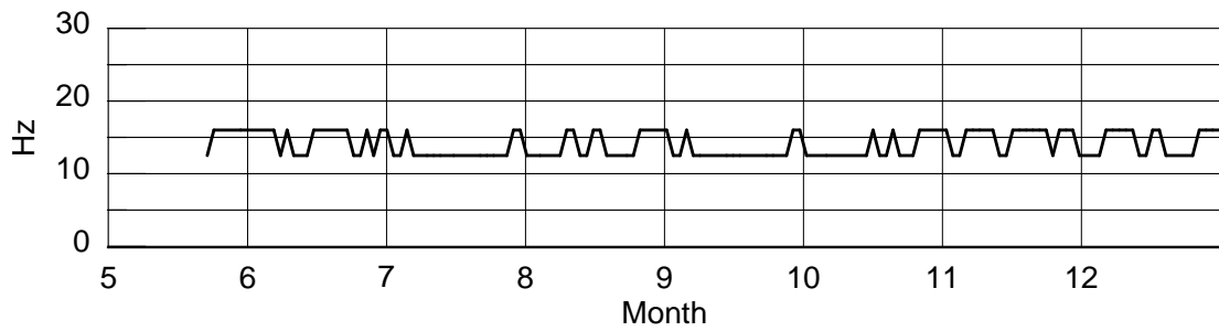
圖 7 台積電測站 108 年 5 月至 12 月頻帶日平均最大值之中心頻率變
