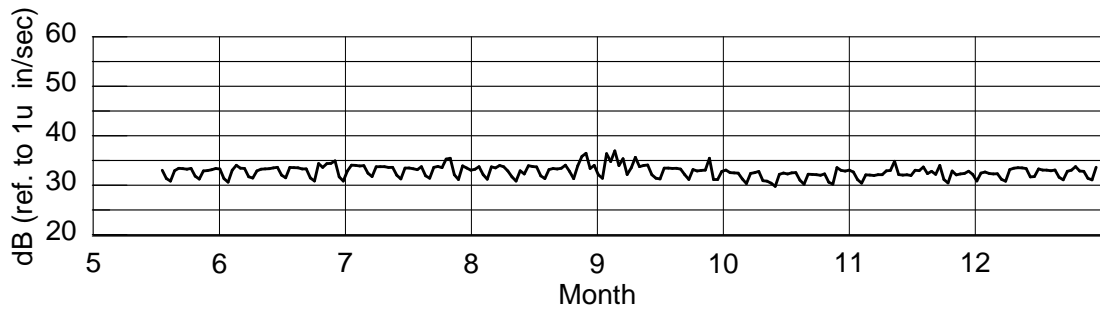
圖 4 台積電測站 108 年 5 月至 12 月頻帶日平均之平均振幅變化圖
