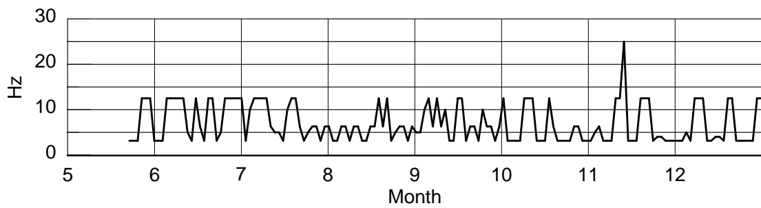
圖 6 景岳測站 108 年 5 月至 12 月頻帶日平均最大值之中心頻率變化
