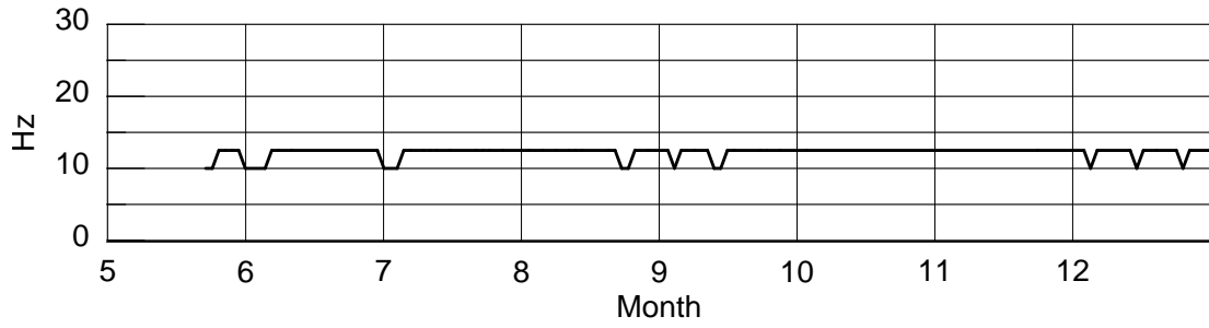
圖 5 橋墩測站 108 年 5 月至 12 月頻帶日平均最大值之中心頻率變化
