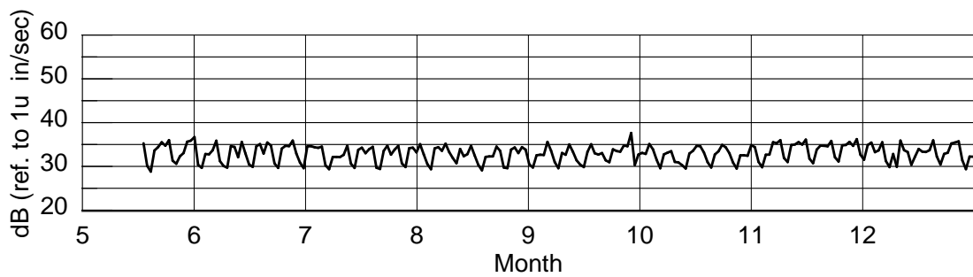
圖 3 景岳測站 108 年 5 月至 12 月頻帶日平均之平均振幅變化圖
