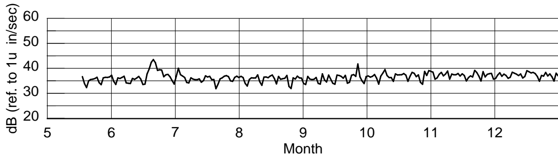
圖 2 橋墩測站 108 年 5 月至 12 月頻帶日平均之平均振幅變化圖
